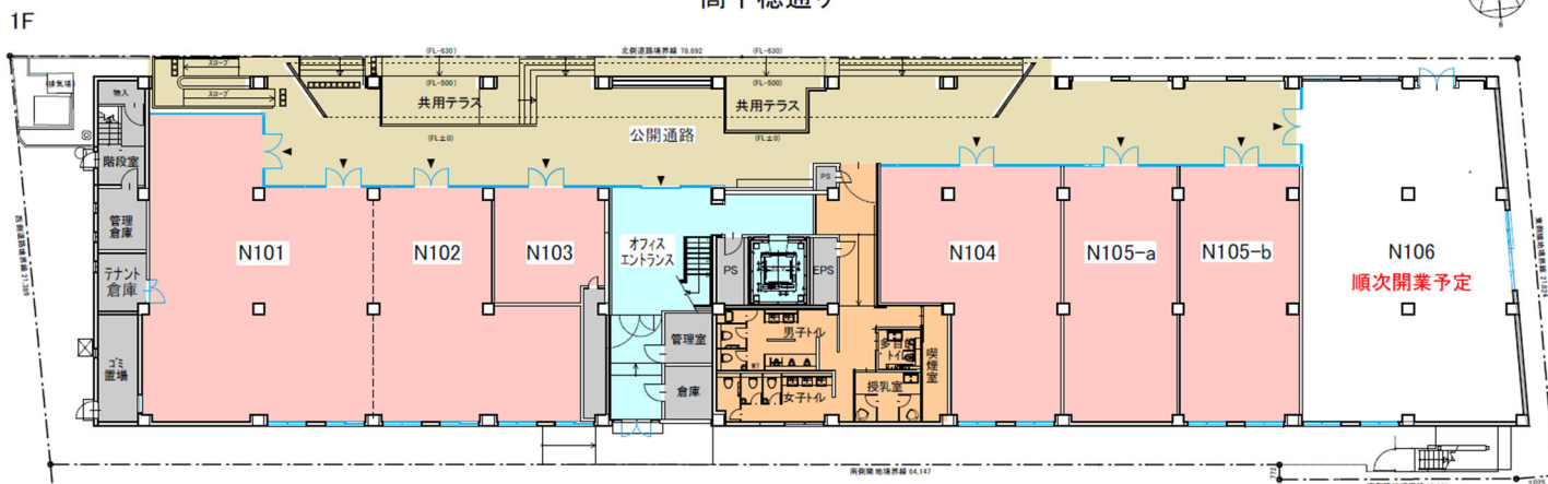
HAROW 高千穂通 1階平面図
