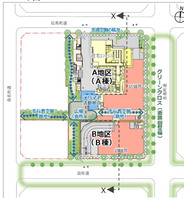
■ 1F 平面
